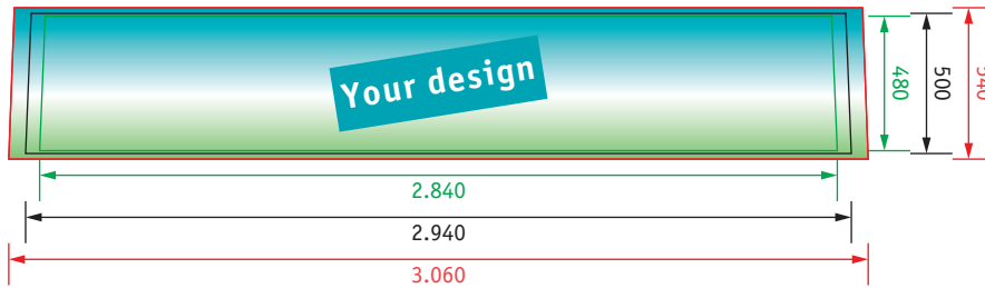
For tent size 6.000 x 3.000
